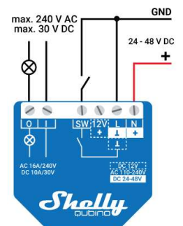
24 V DC
